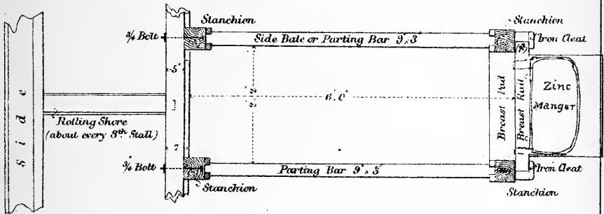
PLAN B.B
